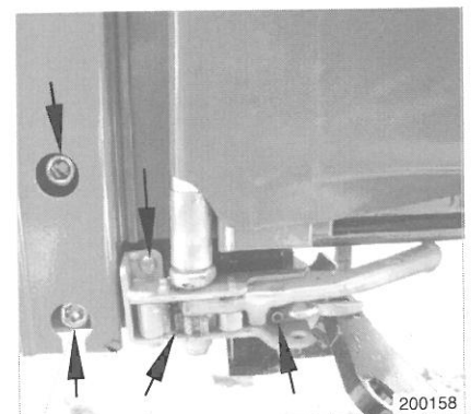
Spanngetriebe hinten
